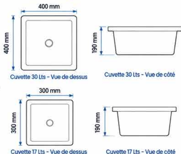
Cuvette 17 Lts - Vue de dessus
